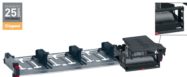
0 321 40 painel equipado com um acessório de gerenciamento de cabos traseiro 0 321 46 + 0 321 41
